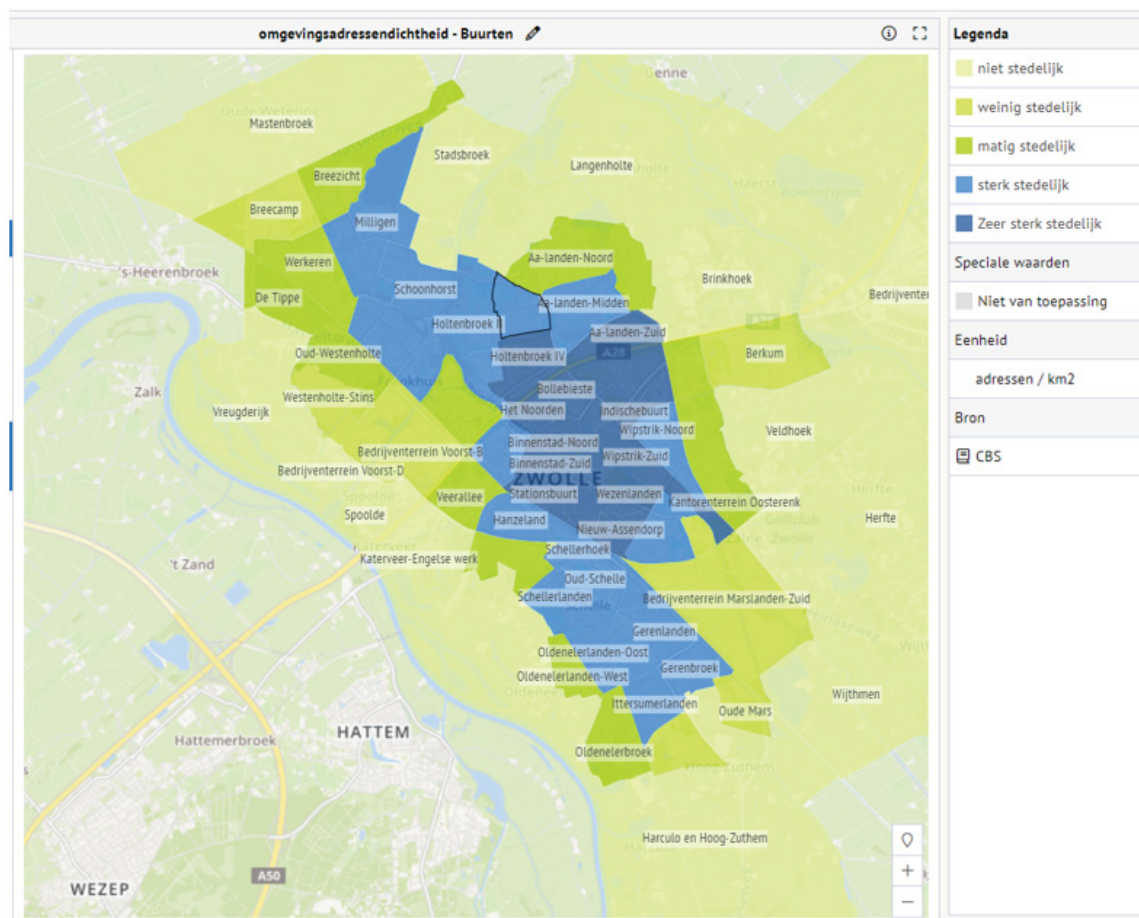
Figuur 1: Omgevingsadressendichtheid
