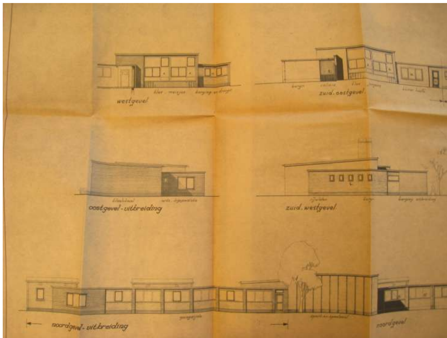
Afb. 17 Kopzijden en (onderaan) zicht op de uitbreiding.
