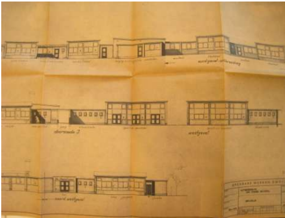
Afb. 14 Lengtegevels en gymzaal (bestaande en nieuwe toestand)
