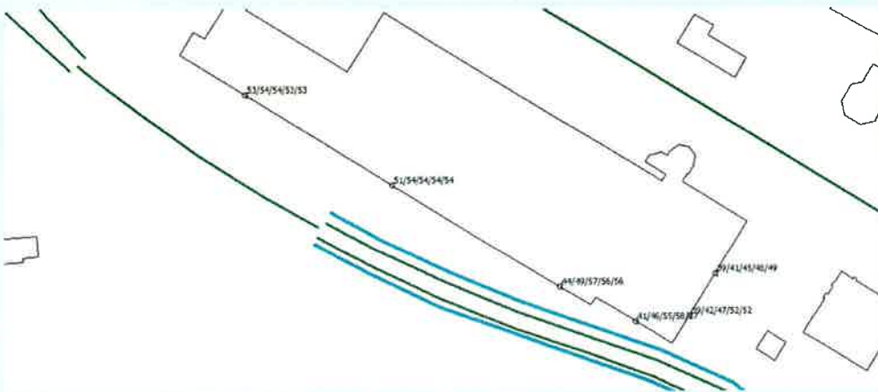
figuur 2: geluidsbelastingen busbaan met barrier 1,1 meter, na aftrek van 5 dB
