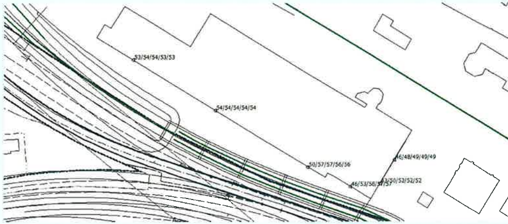
figuur 1: geluidsbelastingen busbaan zonder barrier, na aftrek van 5 dB
