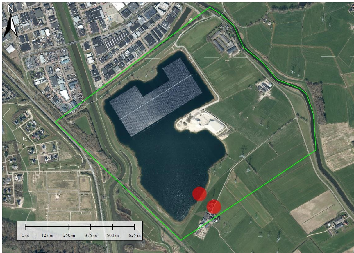
Figuur 17. Het verdachte gebied afwerpmunitie (max. 500 lb, Brits, weergegeven in rood) binnen het projectgebied (weergegeven in groen). Bron satellietbeeld: World Imagery.
